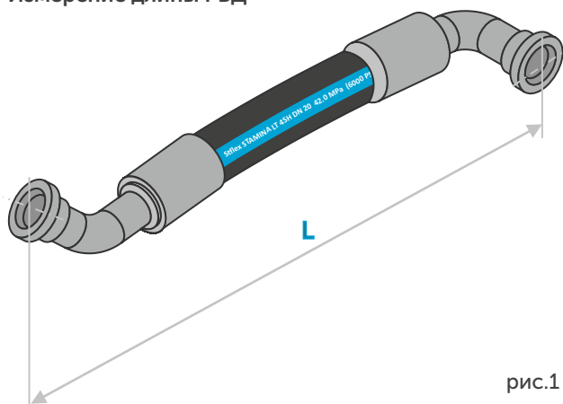
Измерение длины РВД
