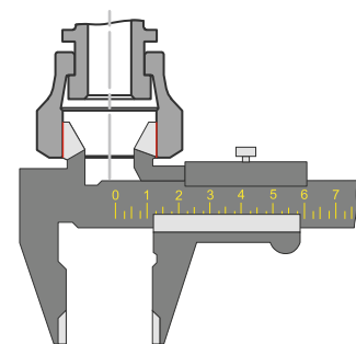
Измерение резьбы по наружному диаметру
