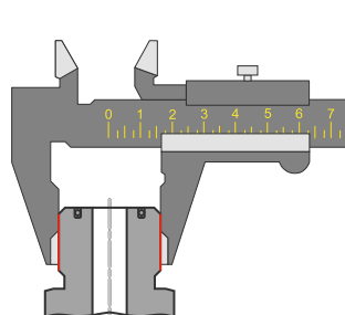
Измерение резьбы по внутреннему диаметру
