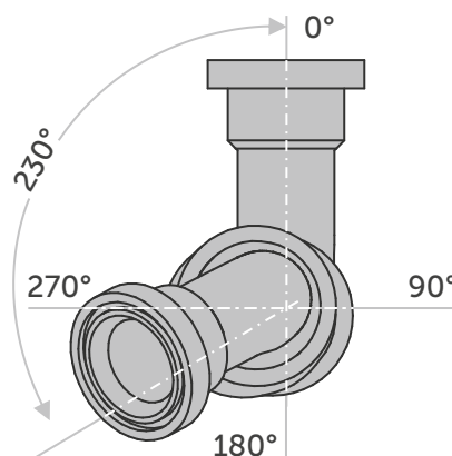
Угол разворота фитингов относительно друг друга
